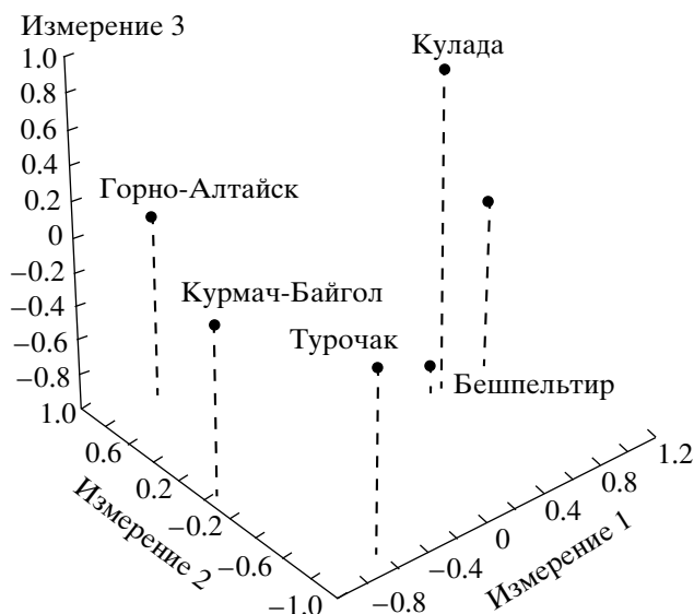
Рис. 3. График многомерного шкалирования Rst-дистанций Слаткина между популяциями алтайцев по частотам YSTR-гаплотипов.
